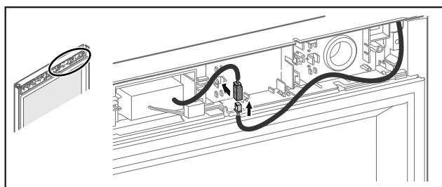
Fig. 37 Glass door
