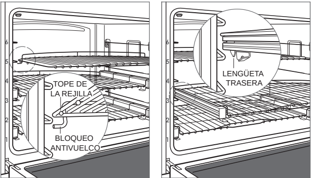
Bloqueo antivuelco para las rejillas del horno Rejilla de máxima extensión
