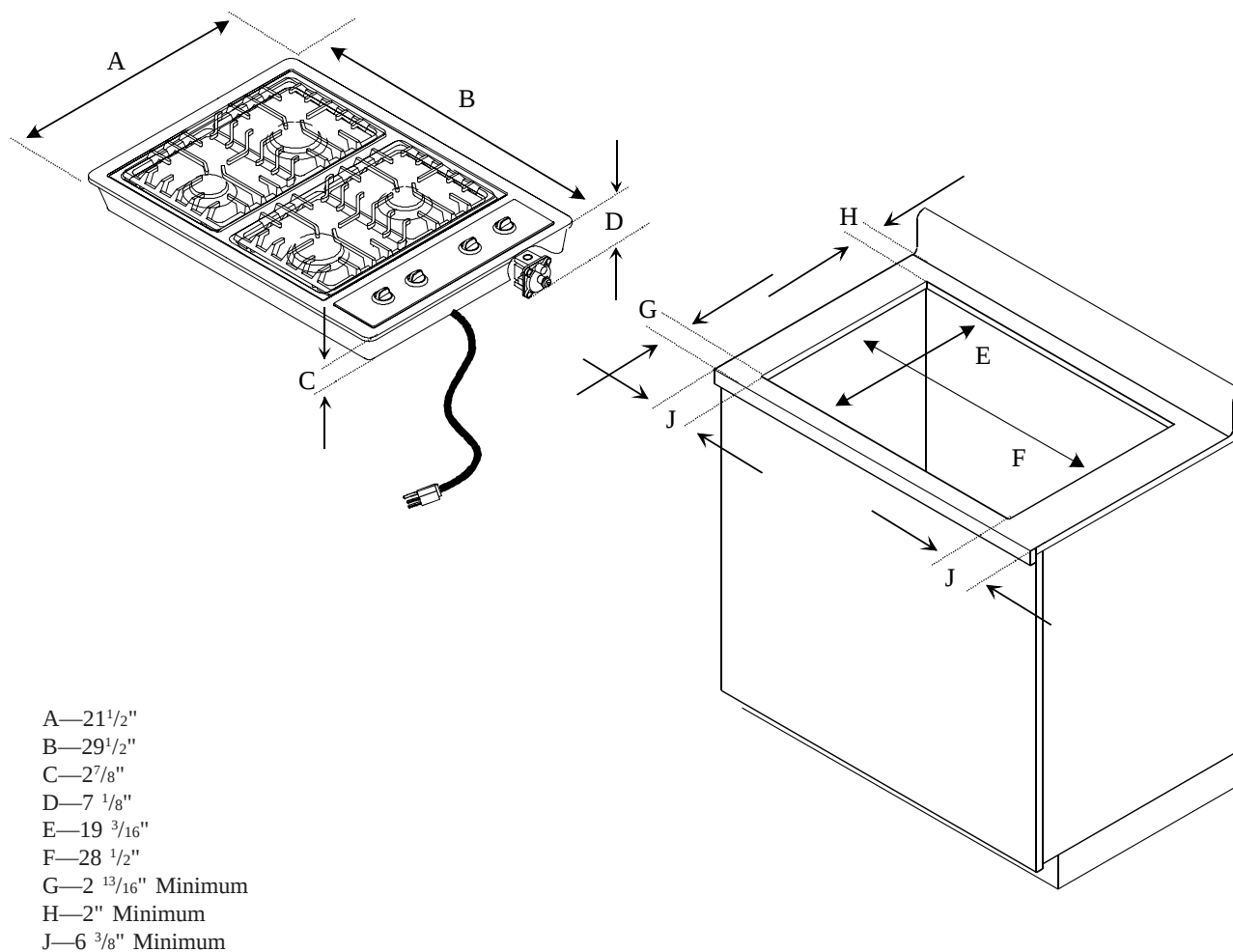
Dimensions de plaque de cuisson
