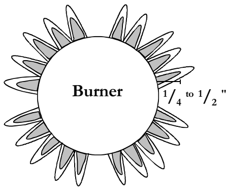
A—Cône interne de \frac{1}{4} à \frac{1}{2} po de long
