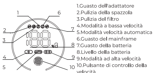
Interruttore
