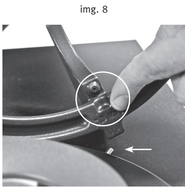
Support de cuisson avec arête de guidage
