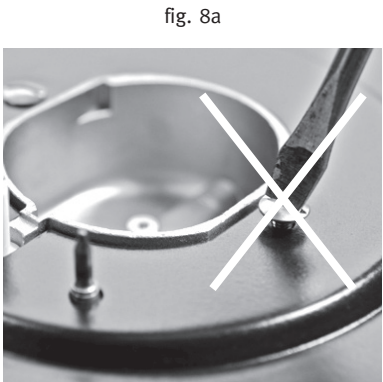
Vite scudo termico
