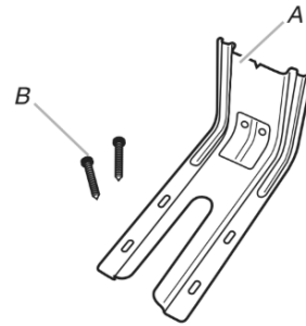
A. Bride antibascullement B. Vis no 12 x 1 5/8 po (4,1 cm) (2)
