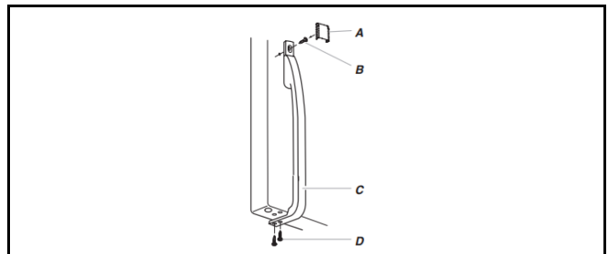
A. Cache-vis
