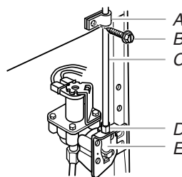
A. Bride du tube B. Vis de bride de tube C. Tube en cuivre
