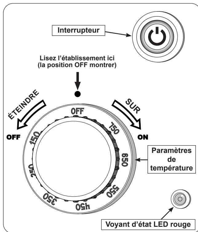
Fig. 36-1 Composants d'allumage
