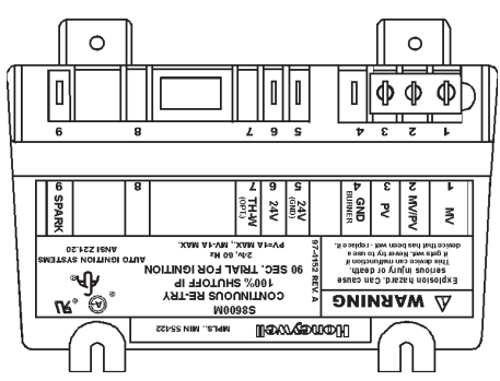
FIGURE 3. MODULE D'ALLUMAGE
