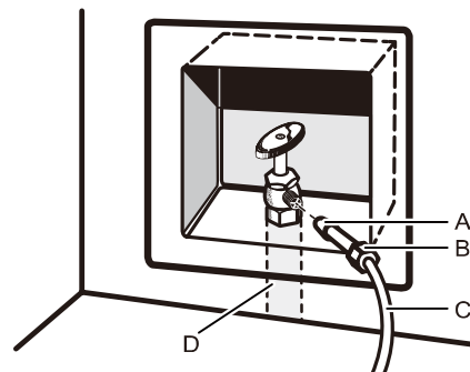
A. Foco B. Tuerca C. Tubería de cobre o PEX (al refrigerador) D. Línea de suministro doméstica (1/2" como mínimo)
