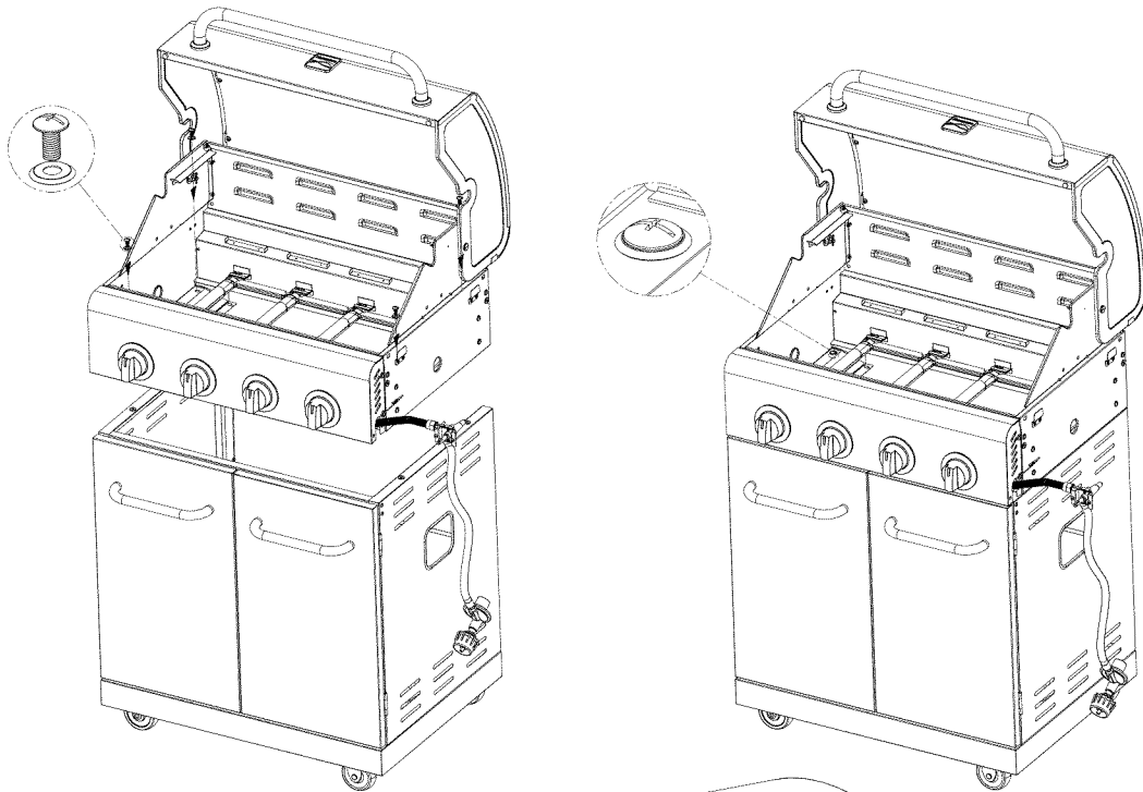
Arandelas de compresión de M6 Cant.:4 us
