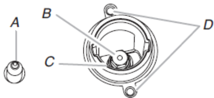
A. Electrodo encendedor B. Tornillo del orificio C. Soporte del tornillo de los orificios D. Tornillos
