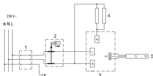
SI. 6: Električna spojna shema
