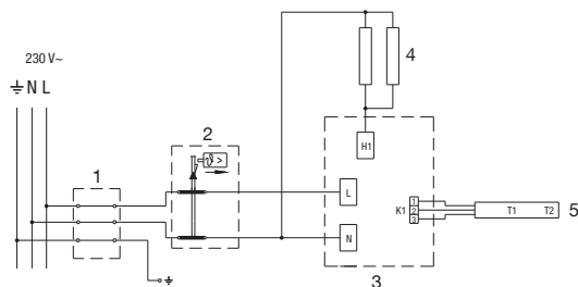
Bild 6: Elektroschaltbild
