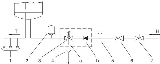
Bild 2: Geschlossenes System (druckfestes System)
