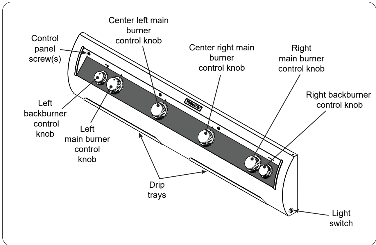
Fig. 35-1 E1060i controls
