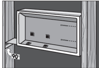
Figura 2 Doble una pata en 90 grados para una instalación a mayor altura y fijela a los puntales.
