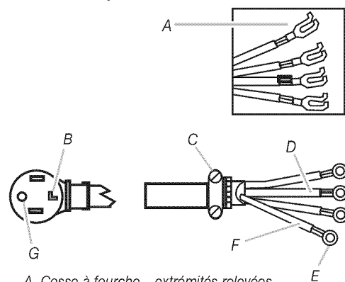
A. Cosse à fourche – extrémités relevées B. Broche neutre C. Serre-câble de \frac{3}{4} " (agrément UL) D. Conducteur neutre (blanc) E. Cosses annulaires F. Conducteur de liaison à la terre G. Broche de liaison à la terre
