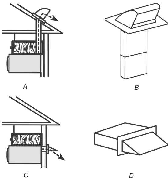
A. Ventilación en el techo
