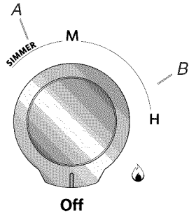
Brûleur à double flamme A. Plage Simmer (mijotage) B. Plage power (puissance)
