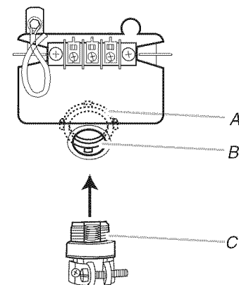
A. Conector del conducto removible B. Orificio debajo de la abertura del bloque de terminal C. Roscas del protector de cables
