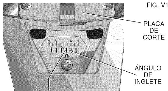
MARCA CENTRAL EN LA ESCALA VERNIER QUEDA ALINEADA CON EL ÁNGULO ENTERO DESEADO EN LA ESCALA DE INGLETE (INGLETE DE 24° A LA DERECHA)
