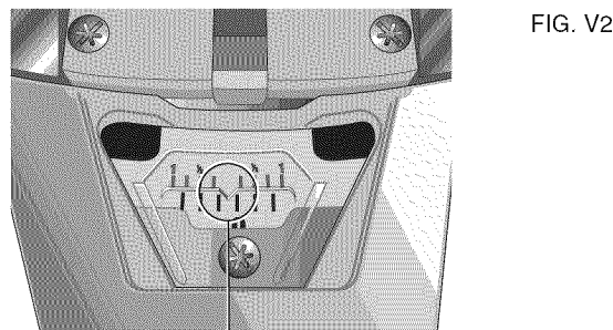
MARCA DE VERNIER A 1/4° QUEDA ALINEADA CON MARCA DE GRADO ENTERO MÁS CERCA EN LA ESCALA DE INGLETE (INGLETE DE 24-1/4° A LA DERECHA)
