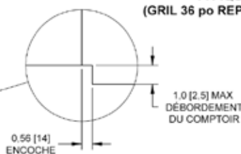
INSTALLATION EN ÎLE TYPIQUE (GRIL 36 po REPRÉSENTÉ)
