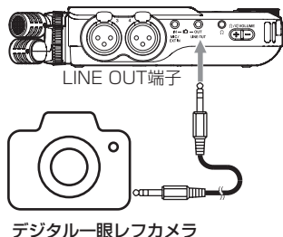
デジタル一眼レフカメラ
