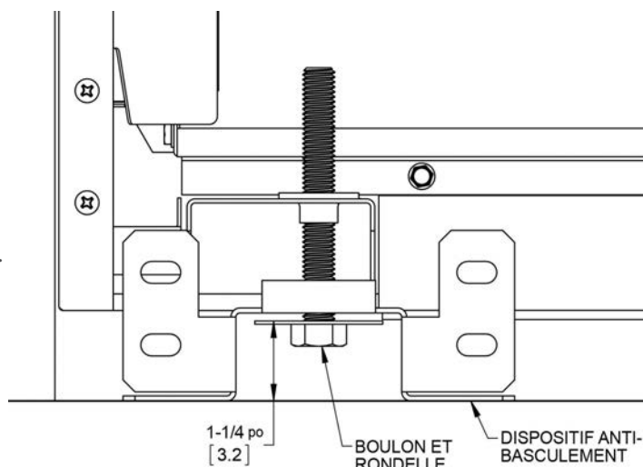
VUE ARRIÈRE
