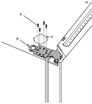
A. 5 mm socket screws B. Top Hinge
