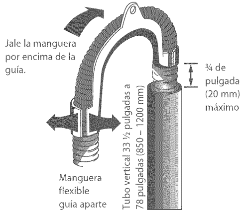
Dibujo 2 Colocar la guía de la manguera de drenaje
