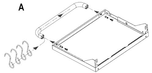
Tornillos de M5x10 Cant.: 2 us Arandelas de seguridad M5 Cant.: 2 us Arandelas de fibra M5 Cant.: 2 us
