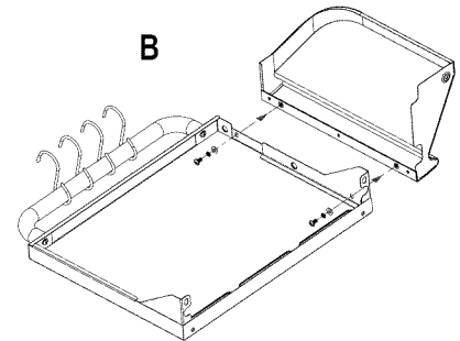
Tornillos de M6x13 Cant.: 4 us Arandelas de seguridad M6 Cant.: 2 us Arandelas de fibra M6 (Dia 16) Cant.: 2 us
