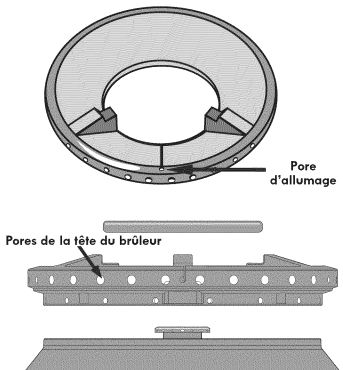
Figure 1- Tête de brûleur G5
