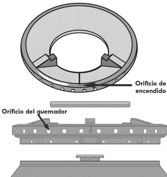
Figura 2- Cabeza de quemador G5
