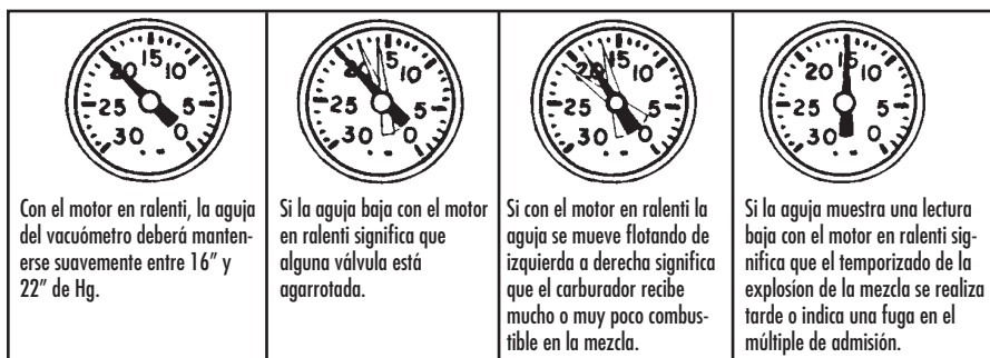
FIGURA 5: LECTURAS DEL VACUÓMETRO
