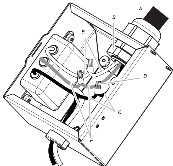
A. Câble d'alimentation électrique du domicile B. Serre-câble (homologation UL ou CSA) C. Conducteurs noirs
