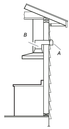
A. Bouche de décharge murale B. Conduit rond de 6" (15,2 cm)
