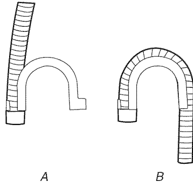
A. Encaje cualquiera de los extremos del molde a la manguera de desagüe en el lugar donde comienza el corrugado. B. Doble la manguera de desagüe sobre el molde y trábela en su lugar.
