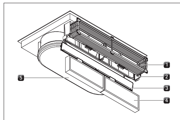
Fig. 5.2 Cooktop extractor recirculation (BIU)
