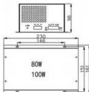
MYJG100W
