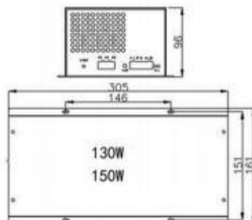
MYJG150W
