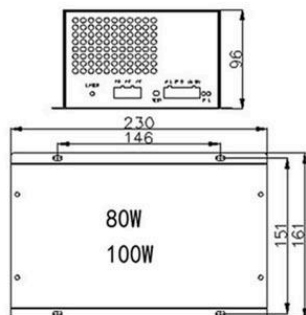
MYJG100W
