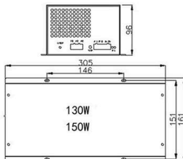
MYJG150W
