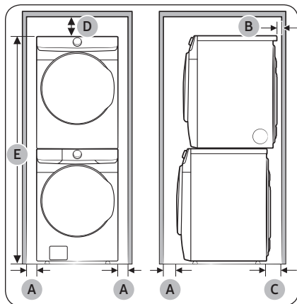
Installation superposée (Modèle : SKK-8K)
