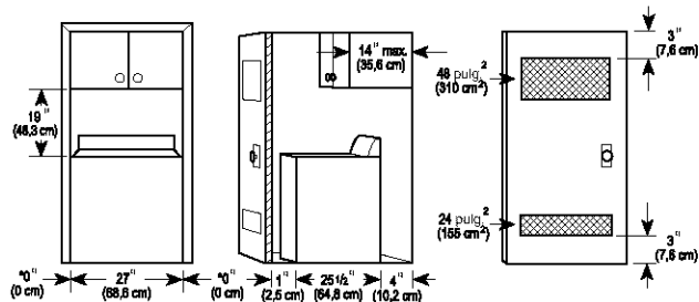
1. Vista de frente 2. Vista lateral 3. Puerta del clóset con orificios de ventilación
