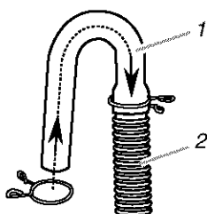
1. Extrémité en col de cygne 2. Tuyau de vidange
