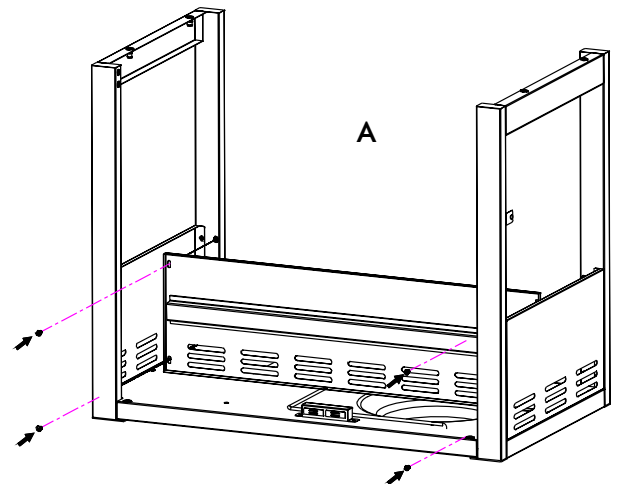
Assemblage du panneau droit
