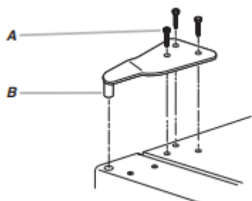
A. Vis de charnière à tête hexagonale de 5/16 po
