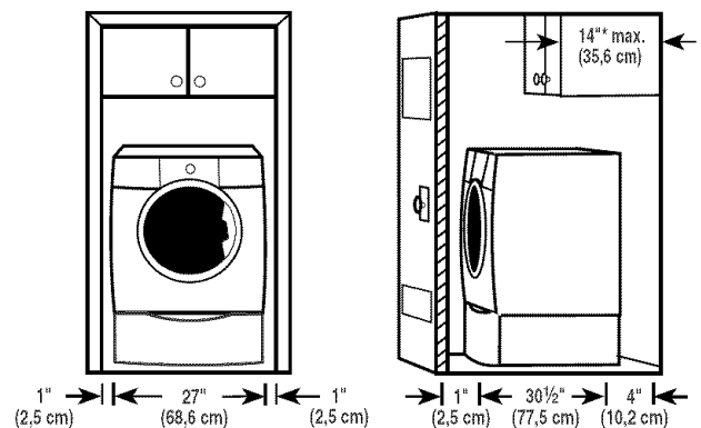
A. Encastrément B. Vue latérale - placard ou endroit exigü
