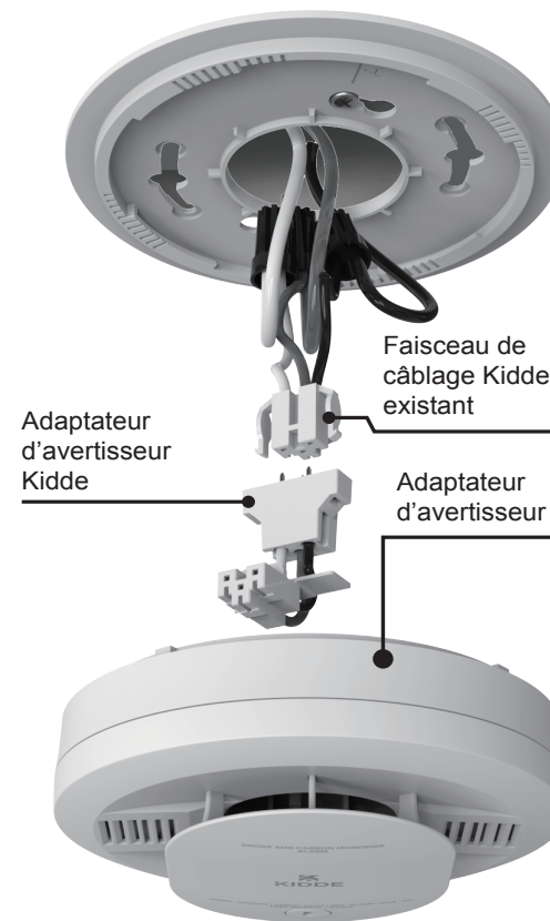
Figure 2 : connexion de l'adaptateur à l'ancien faisceau
