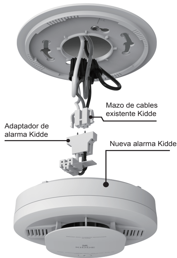
Figura 2: Adaptador conectado al mazo de cables antiguo
