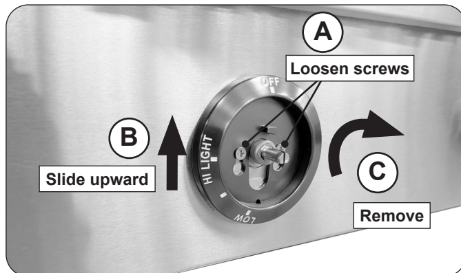
Fig. 40-2 Remove bezels
