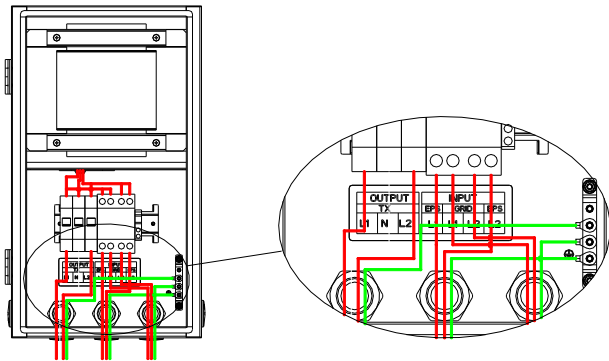
Fig 1.5 ATS-5K Wiring Diagram
