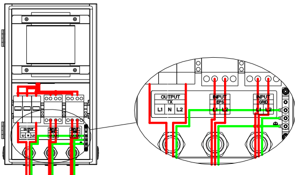
Fig 1.6 ATS-11.4K Wiring Diagram
