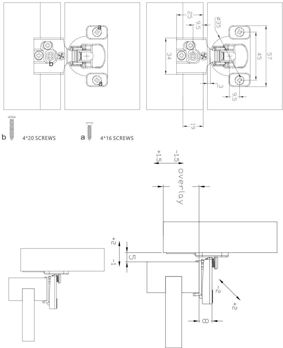
MARCO FRONTAL CON CIERRE SUAVE AJUSTABLE DE CUATRO PUNTAS \varnothing 35(2D) BISAGRAS
