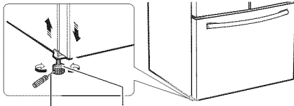
Tournevis à tête plate (-) Molette
