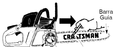
Rueda de Ajuste Perilla de la barra Destornillador
