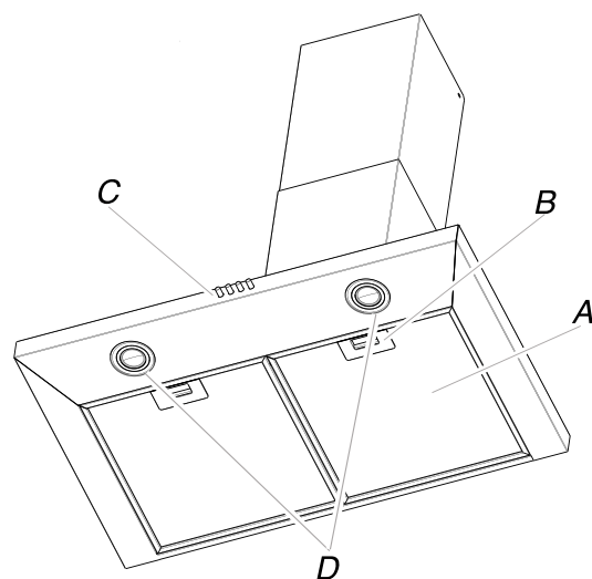
A. Filtre à graisse B. Poignée du filtre à graisse C. Commandes du ventilateur et de l'éclairage D. Lampes DEL
