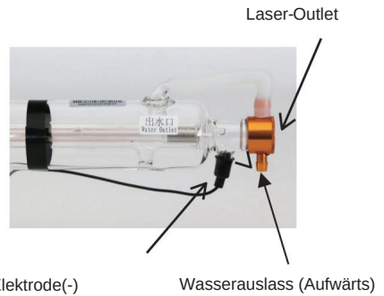
Negative Elektrode(-)
