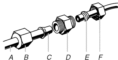
A. Tube vers réfrigérateur B. Écrou (fourni) C. Renflement D. Raccord (fourni) E. Virole (à acheter) F. Écrou (à acheter)
