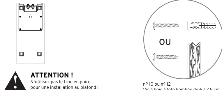
FIGURE 4 MONTAGE MURAL DES ENCEINTES SURROUND
