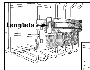
Tope de bloqueo de Lengüeta
