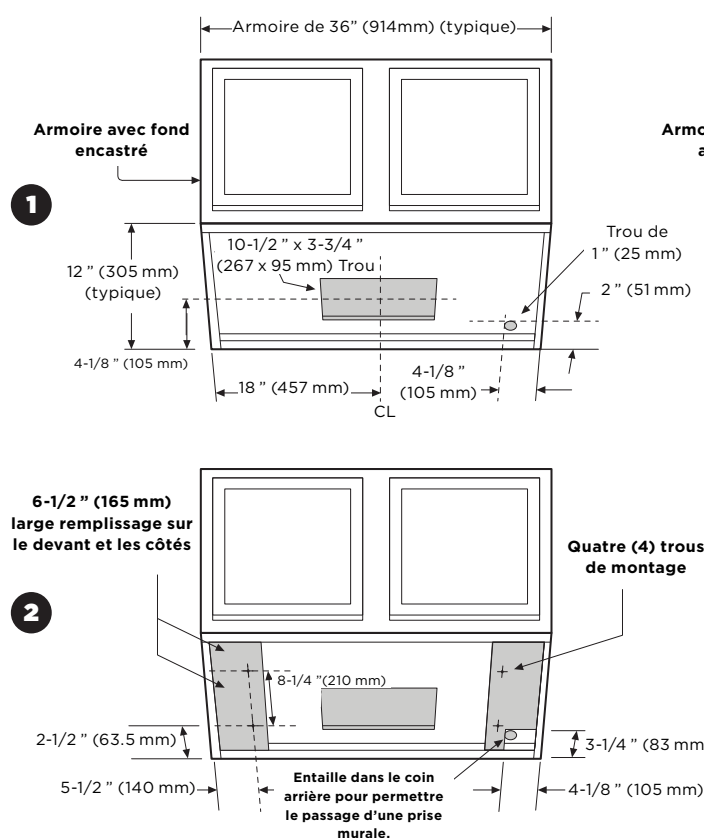
Armoire avec fond encastré
