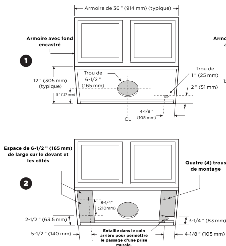
Armoire avec fond encastré
