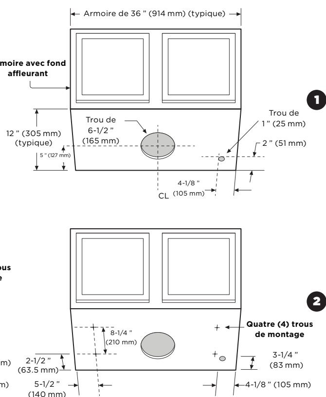
Armoire avec fond affleurant
